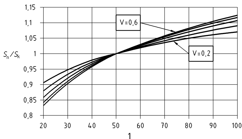
Figure D.1 Ajustement de la charge de neige sur le sol en fonction de la période de retour
