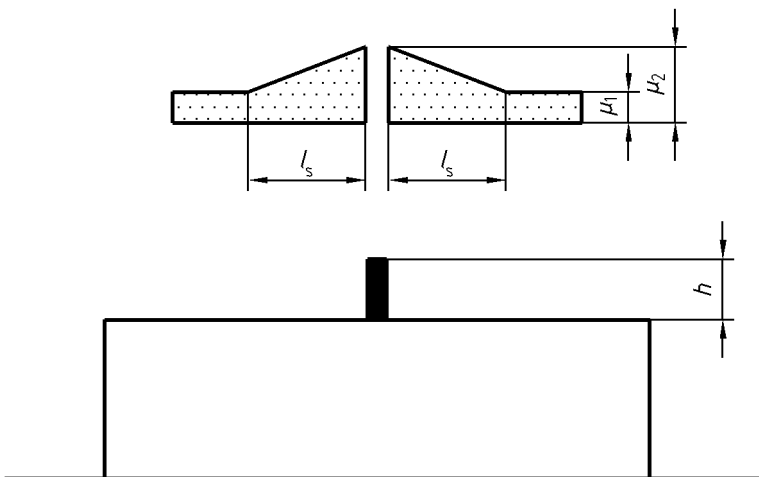
Figure 6.1 Coefficients de forme pour charge de neige aux saillies et obstacles
